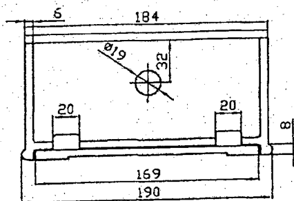
CORTE C-D
